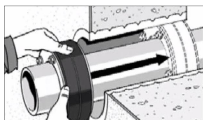
Monteres som vist her – mot våt side
