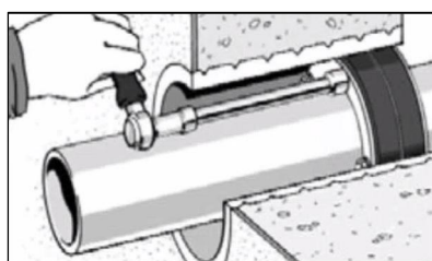
Muttere tilspennes kryssvis
