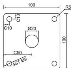
DETALJ A
