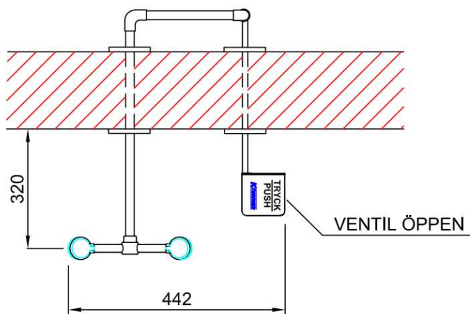
SEKTION A - A
